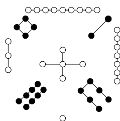
圖 2.2 洛書
