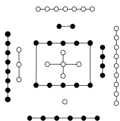
圖 2.1 河圖
