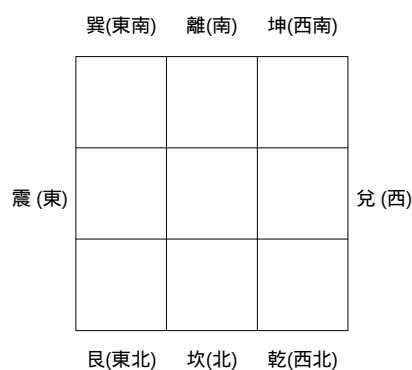
圖 3.12 九宮方位圖
