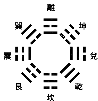
圖 2.5 後天八卦
