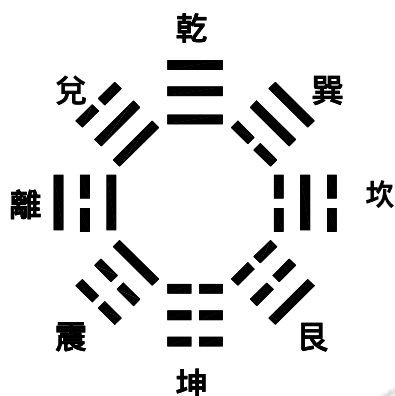
圖 2.4 先天八卦
